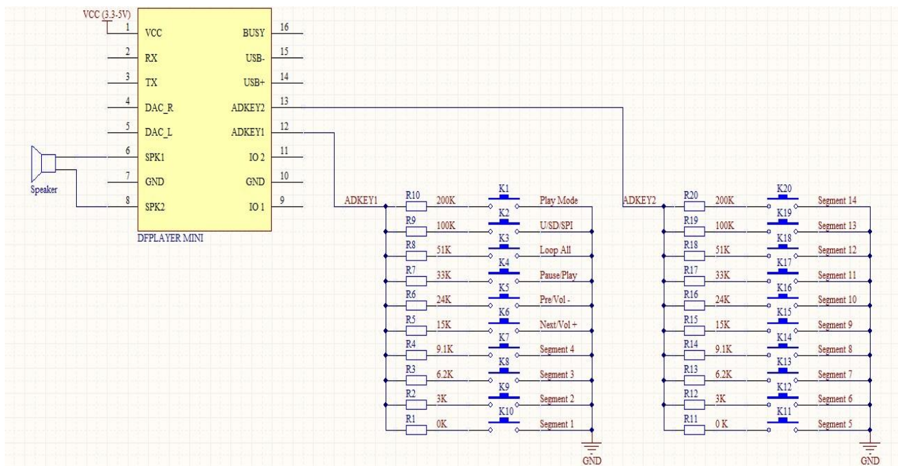
איור 3 : שימוש בלחצנים עבור כניסות ADKEY2 ו ADKEY1
