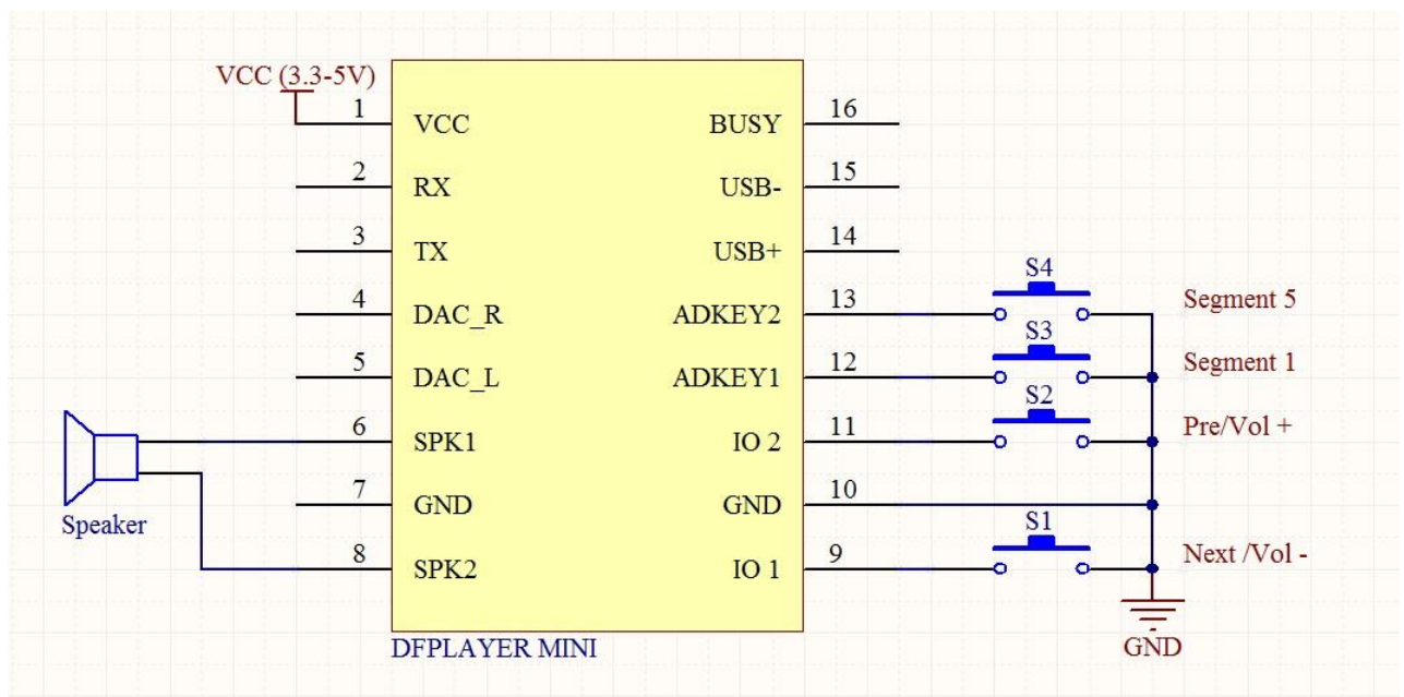
איור 4 : שימוש בלחצני ADKEY2 , ADKEY1 בנוסף לכניסות IO1 ,IO2
